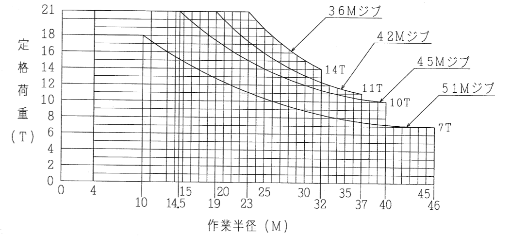
性能線図
