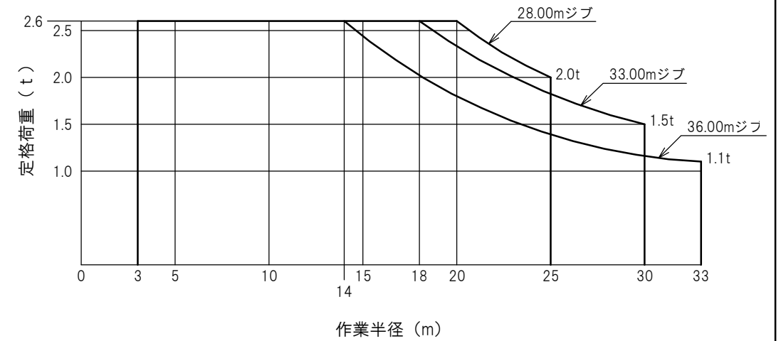
定格荷重線図
