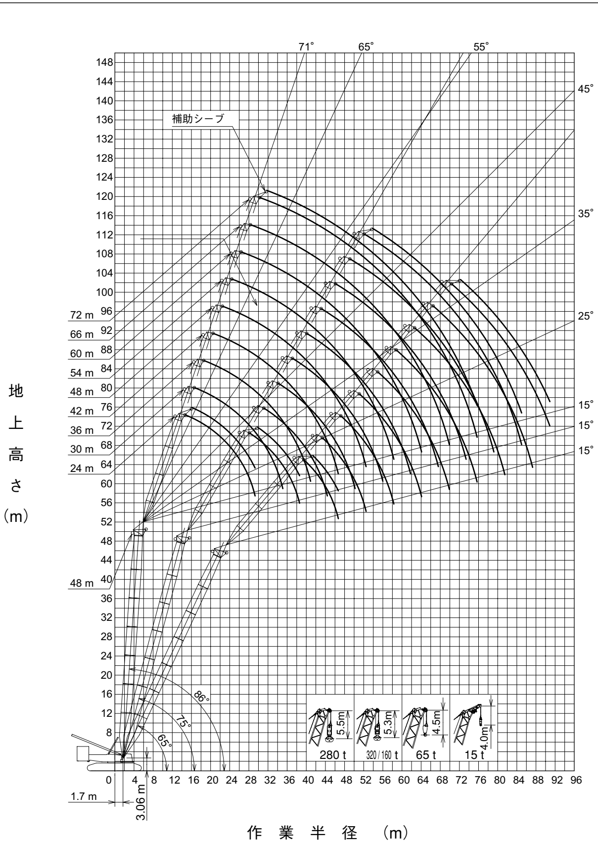
■作業範囲図：48 m タワー+ジブ
