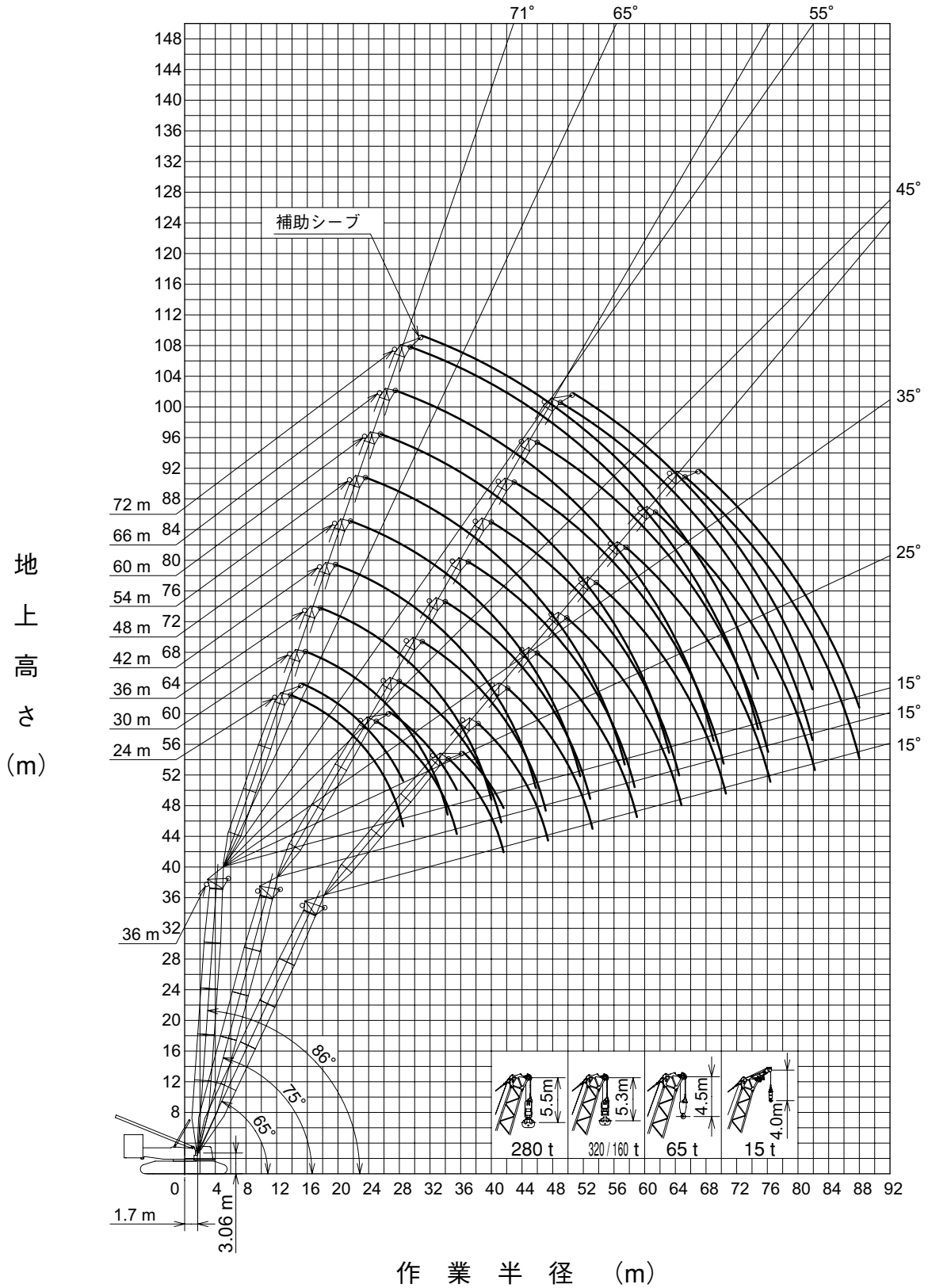
■作業範囲図：36 m タワー+ジブ
