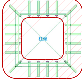
柱脚折曲げ定着表示
