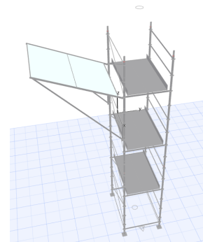
「2300」サイズ
