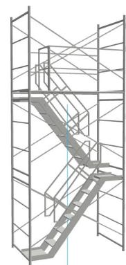
全閉鎖
