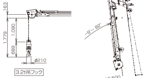
2段パワーチルトジブ
