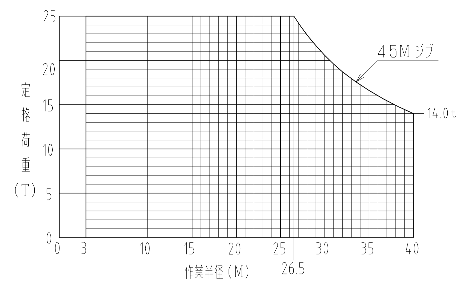
定格荷重線図
