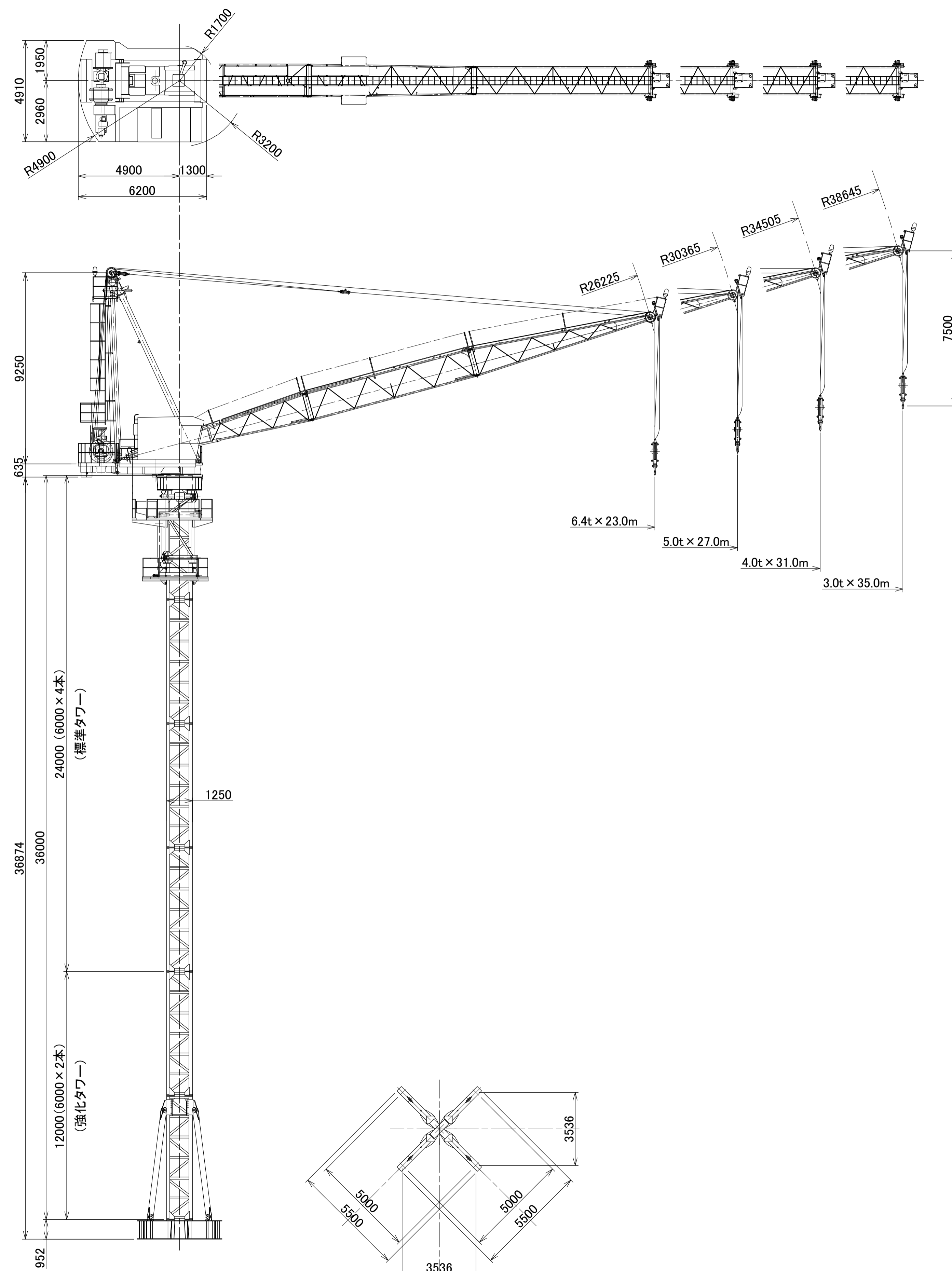
台座平面図
