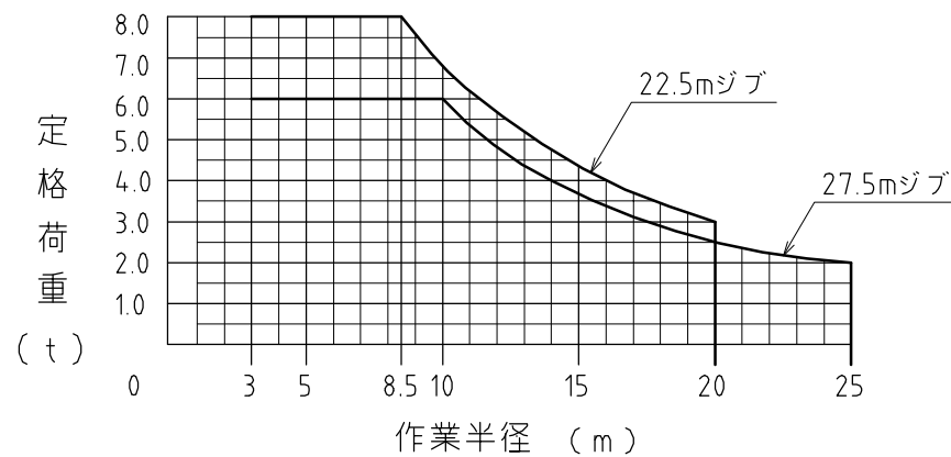
定格荷重線図 (4本掛け)
