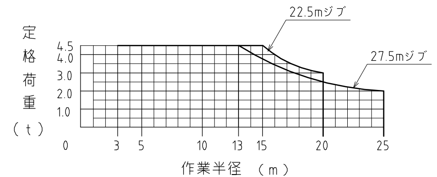
定格荷重線図 (2本掛け)
